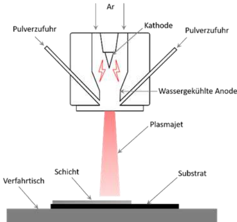
Schematische Darstellung des Kaltplasmaspritzsystems (Cold Plasma Spraying - CoPla)
