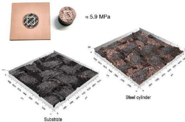
Ansicht einer Cu-Beschichtung auf CFK-Material nach dem Stempelabriss, mit entsprechenden Konfokal-Mikroskopie-Aufnahmen
