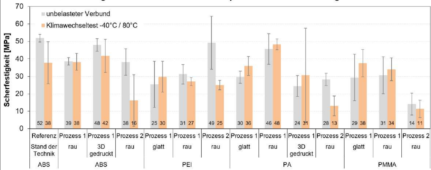
Scherfestigkeit an mit Chemisch Nickel metallisierten ABS-, PEI-, PA-, PMMA-Substraten, im Vergleich zu ABS nach Stand der Technik
