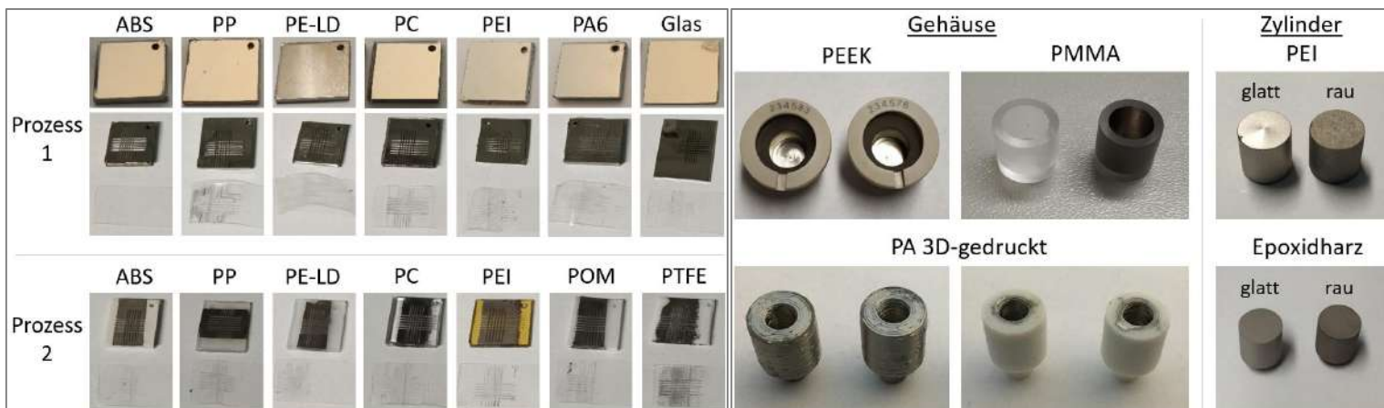
Metallisierte Flachsubstrate (glatt) nach Prozess 1 & 2; Gitterschnitt 3D-Bauteile: Metallisierung der Außen- / Innenkontur
