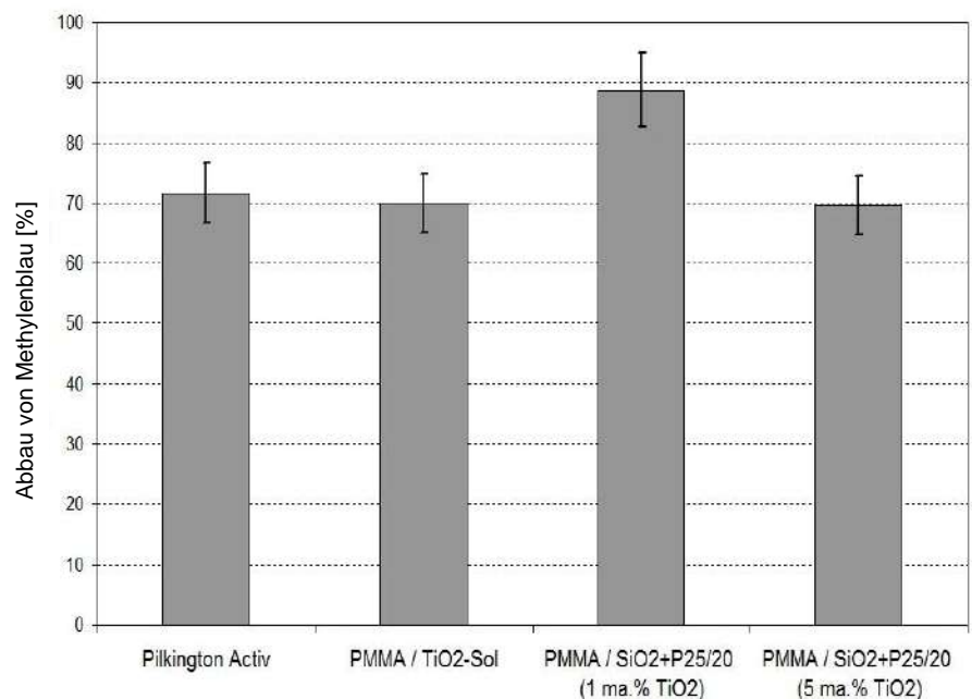
Photokatalytische Aktivität von bei INNOVENT entwickelten TiO x -Solten auf PMMA im Vergleich zu einem kommerziell erhältlichen mit TiO x beschichtetem Glas (Pilkington Activ)
